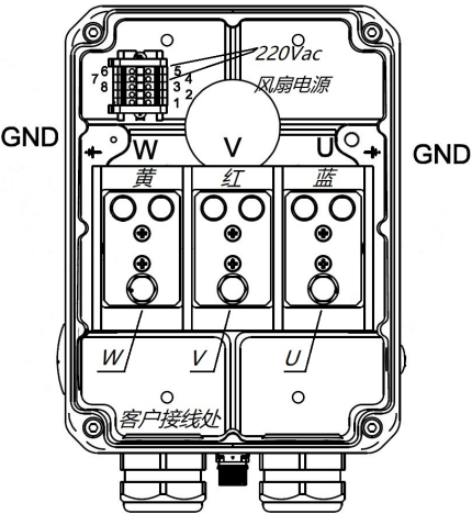
● U318F 风冷电机接线端子示意图
