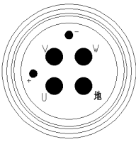
M40 电源插座 (30Arms < 额定电流≤ 60Arm)
