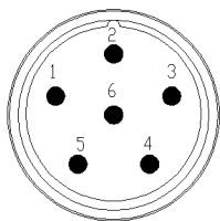
M23 电源插座 ( 额定电流≤ 30Arms)
