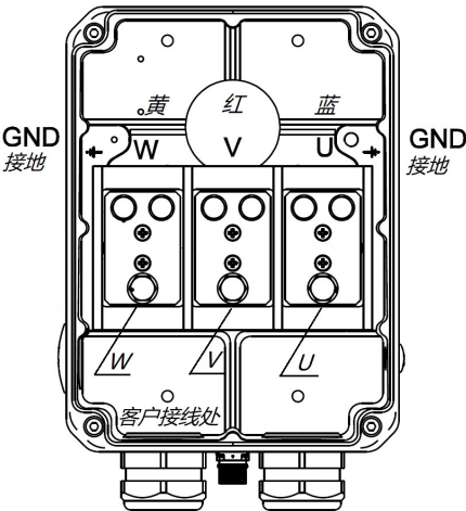
● U318C 液冷电机接线端子示意图
