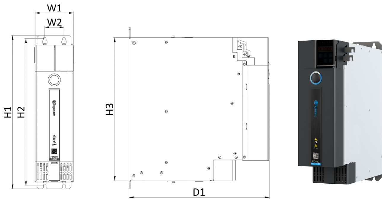
外形尺寸 Overall Dimensions
