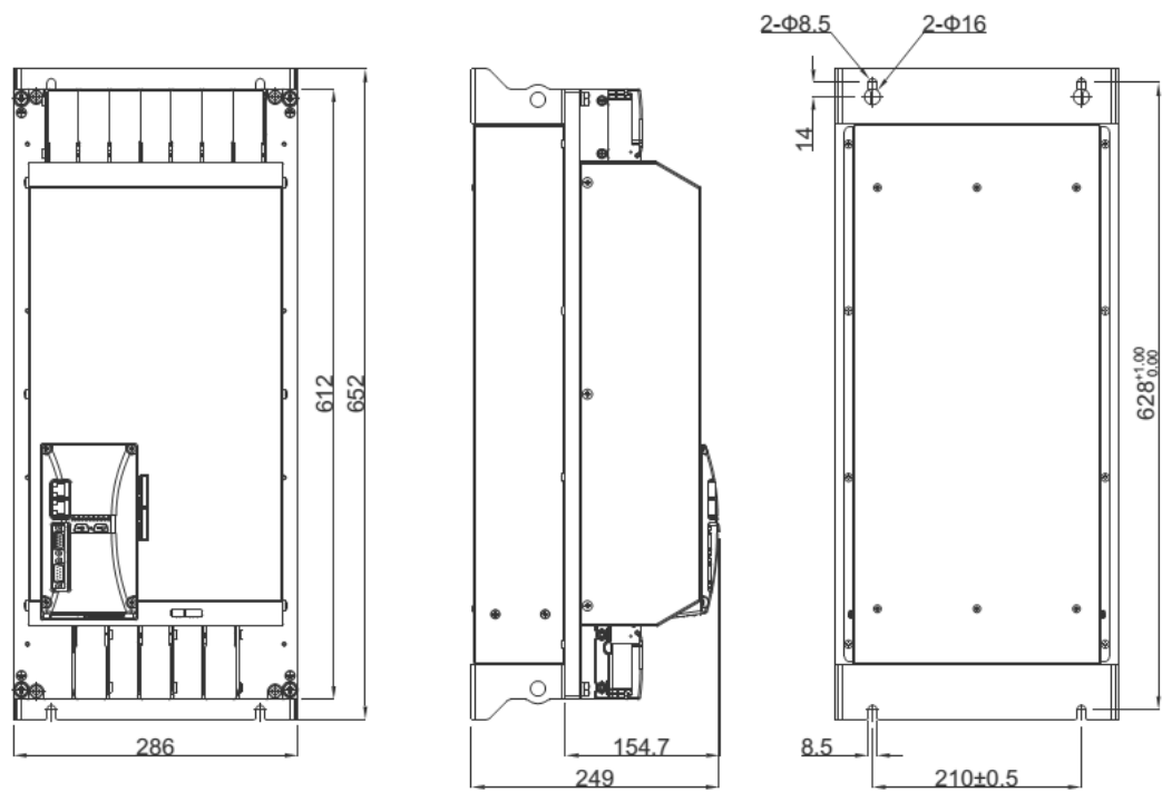
AxN Size5 系列驱动器外形尺寸
