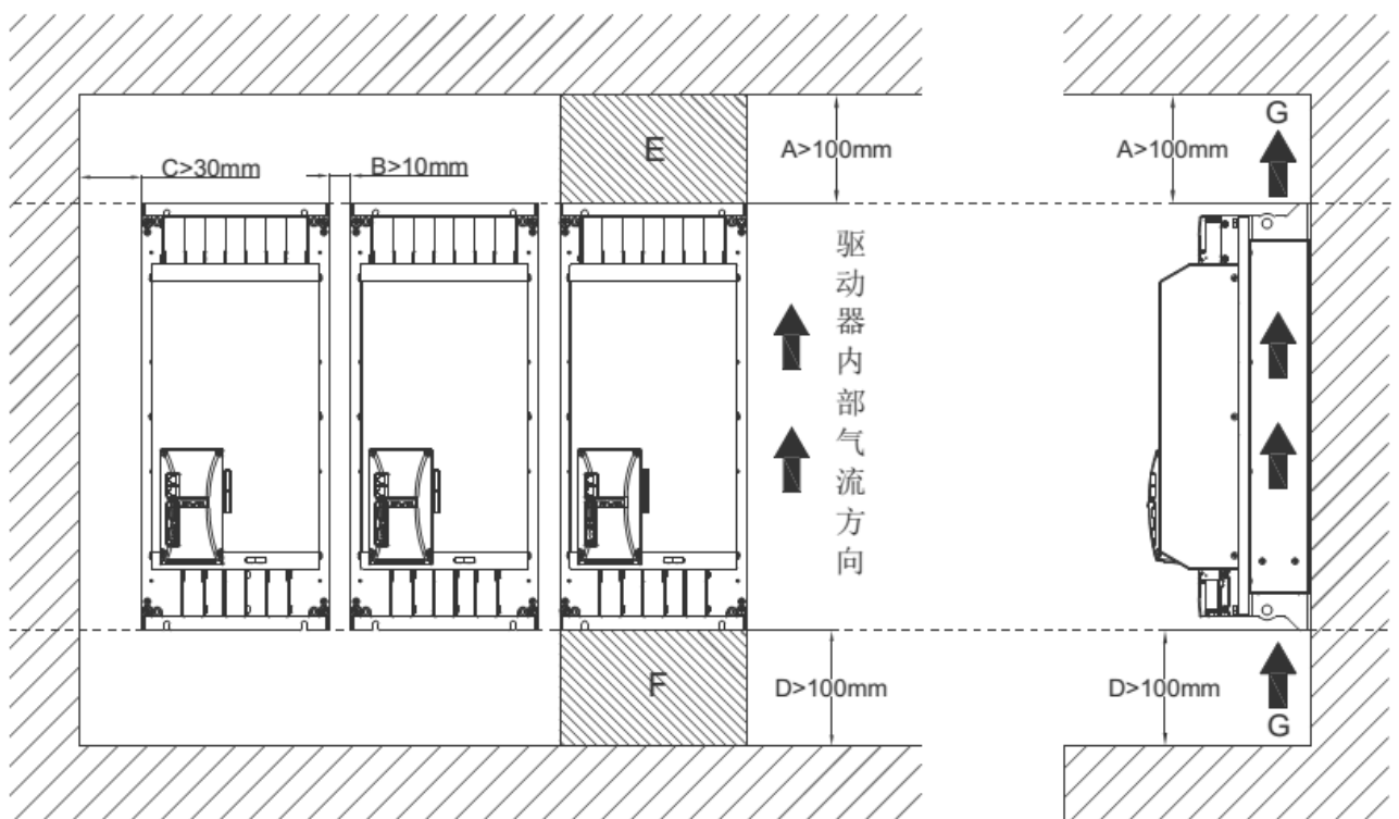
AxN Size5 系列驱动器安装间隙
