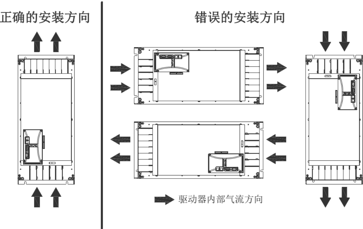
AxN Size5 系列驱动器安装方向
